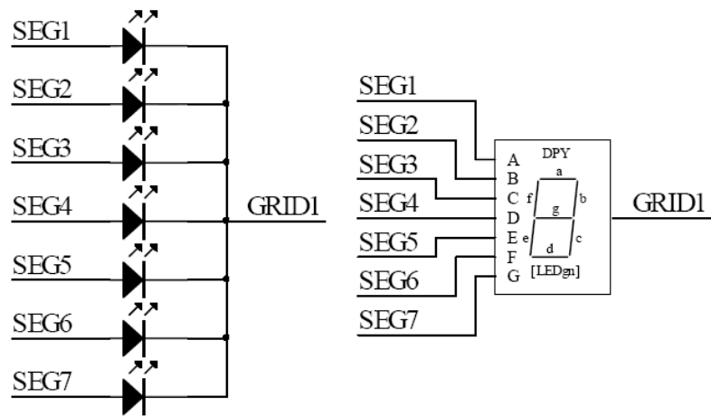
图8、共阴数码管
