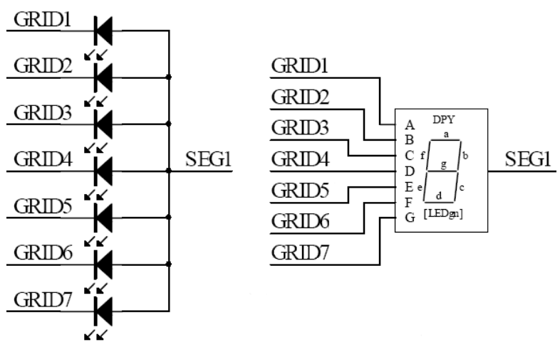
图9、共阳数码管
