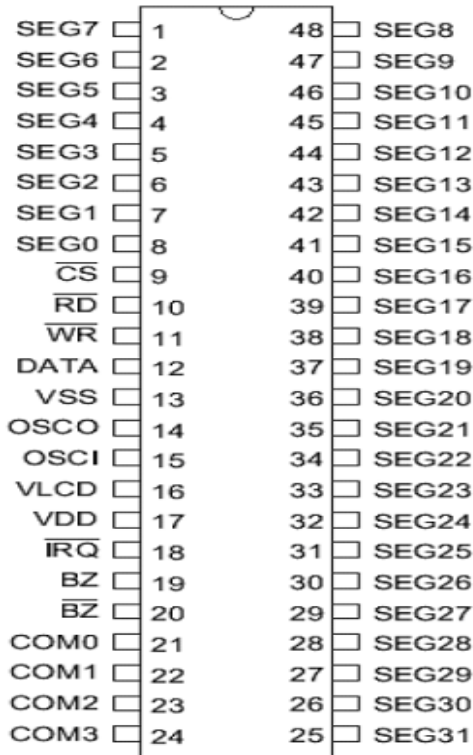
SSOP48
